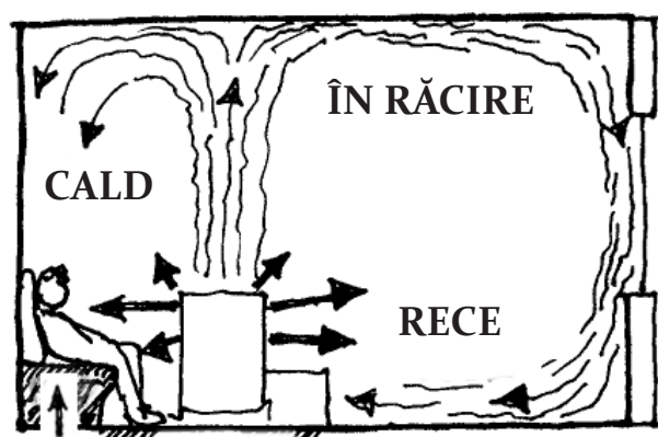
Sobă-rachetă
