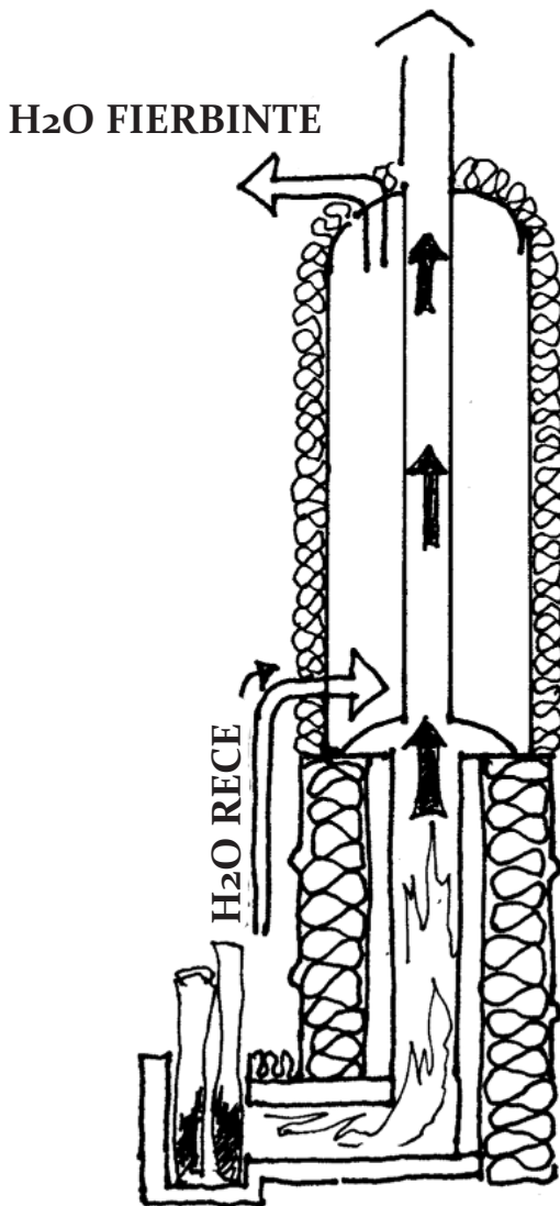
Ideea generală de montare a unui boiler deasupra conductei de căldură ascendentă a unei sobe-rachetă.
